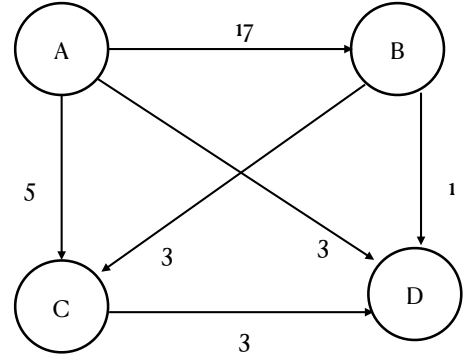
(b) V-IMDC-u counterexample (DAG)
