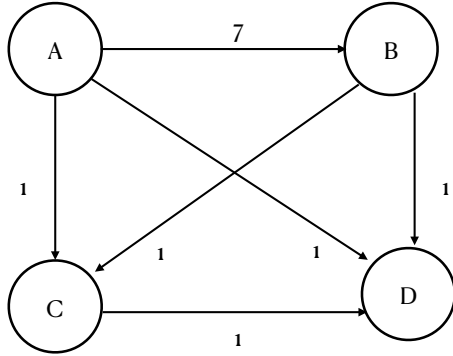
(a) P-IMDC-u counterexample (DAG)
